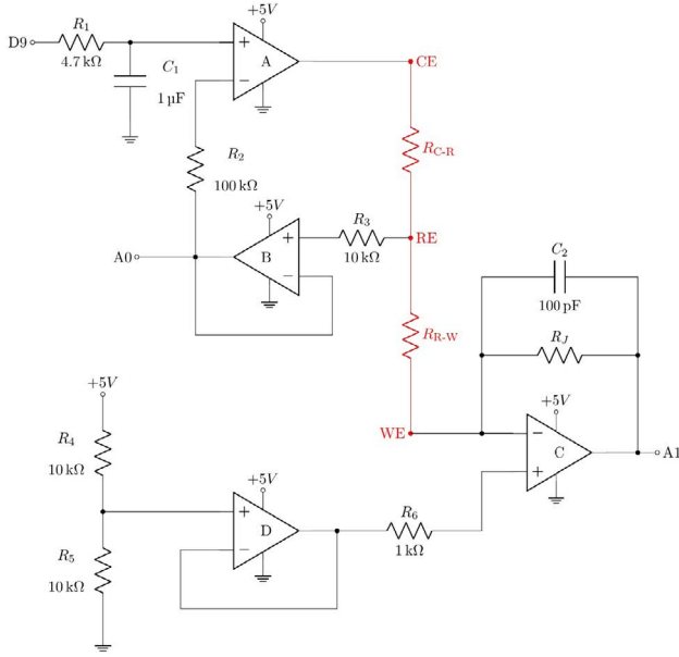
Fig. 1. Diagrama electrónico del circuito de control propuesto.
