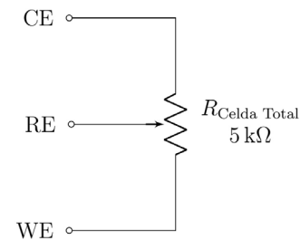
Fig. 3. Diagrama de conexión de un potenciómetro para simular una celda electroquímica con un determinado factor resistivo.
