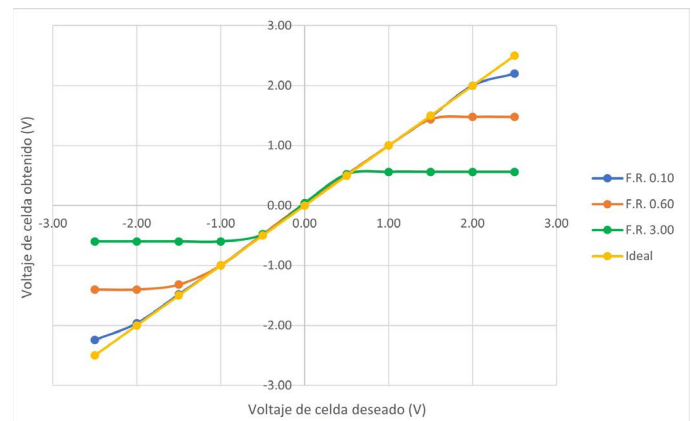
Fig. 4. Comparación entre los voltajes de celda deseados y los obtenidos para tres diferentes valores de factor resistivo y una resistencia de celda total de 5 \text{ k}\Omega .
