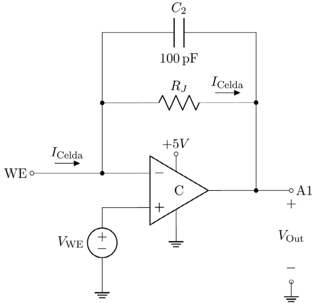
Fig. 2. Circuito simplificado del amplificador seguidor de corriente.
