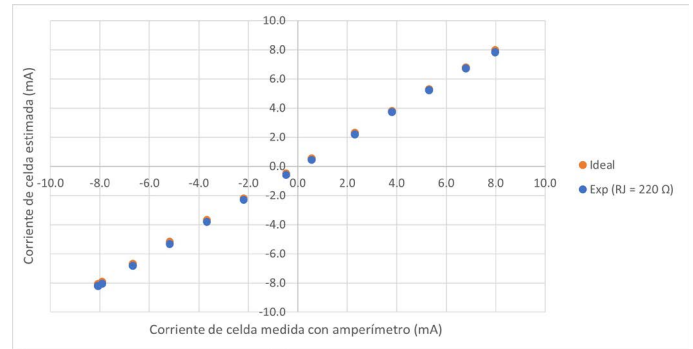
Fig. 8. Corriente de celda medida con amperímetro (mA) contra corriente de celda estimada (mA) con el potencióstato para una resistencia de celda total de 220 \Omega , para 16 diferentes valores de ancho de pulso aplicados a la señal PWM.
