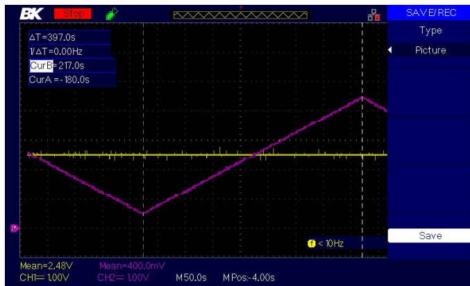
Fig. 7. Oscilograma que muestra el voltaje de los electrodos de referencia (morado) y trabajo (amarillo) durante un barrido de -2 V a +2 V en el voltaje de celda. Los cursores (línea punteada) se utilizan para medir la velocidad de barrido experimental.
