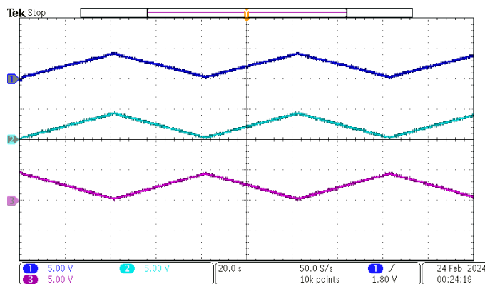
Fig. 6. Oscilograma que muestra: 1) el voltaje obtenido a partir de la señal PWM; 2) el voltaje del electrodo de referencia; y 3) el voltaje de salida del seguidor de corriente, para un barrido de voltajes de celda entre -2\text{ V} y +2\text{ V} con factor resistivo de 0.10, resistencia total de celda de 5\text{ k}\Omega , y R_j de 4.7\text{ k}\Omega .
