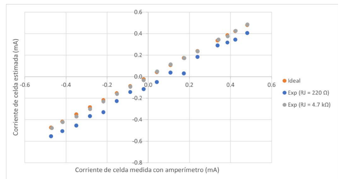
Fig. 10. Corriente de celda medida con amperímetro (mA) contra corriente de celda estimada (mA) con el potencióstato para una resistencia de celda total de 5.1 k\Omega , para 16 diferentes valores de ancho de pulso aplicados a la señal PWM.
