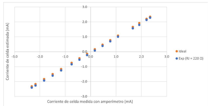
Fig. 9. Corriente de celda medida con amperímetro (mA) contra corriente de celda estimada (mA) con el potencióstato para una resistencia de celda total de 1 k\Omega , para 16 diferentes valores de ancho de pulso aplicados a la señal PWM.
