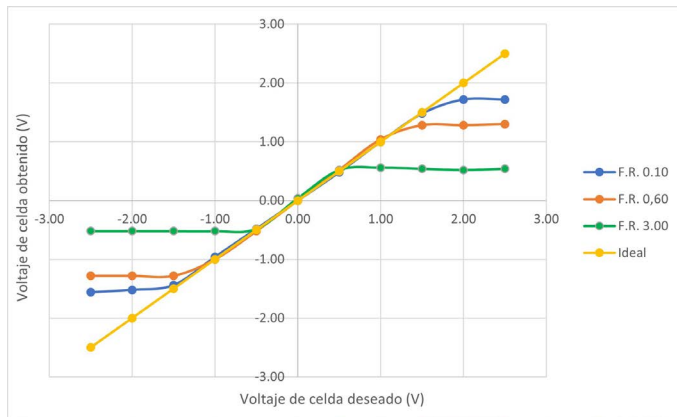
Fig. 5. Comparación entre los voltajes de celda deseados y los obtenidos para tres diferentes valores de factor resistivo y una resistencia de celda total de 500\ \Omega .
